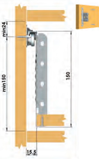
• Min. drawer height
